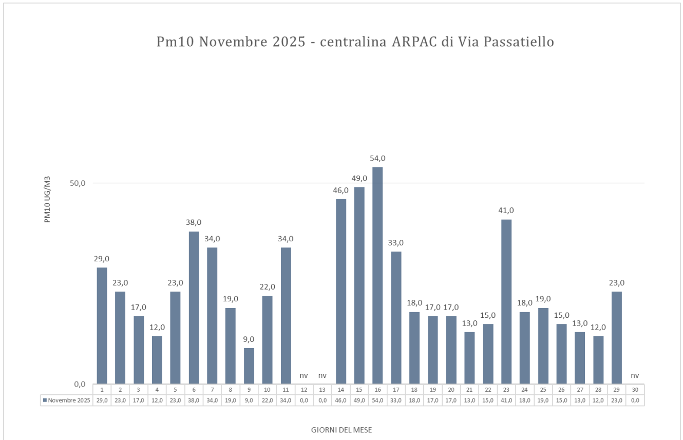
Grafico 1. Andamento polveri sottili PM10 mese di novembre 2025.
