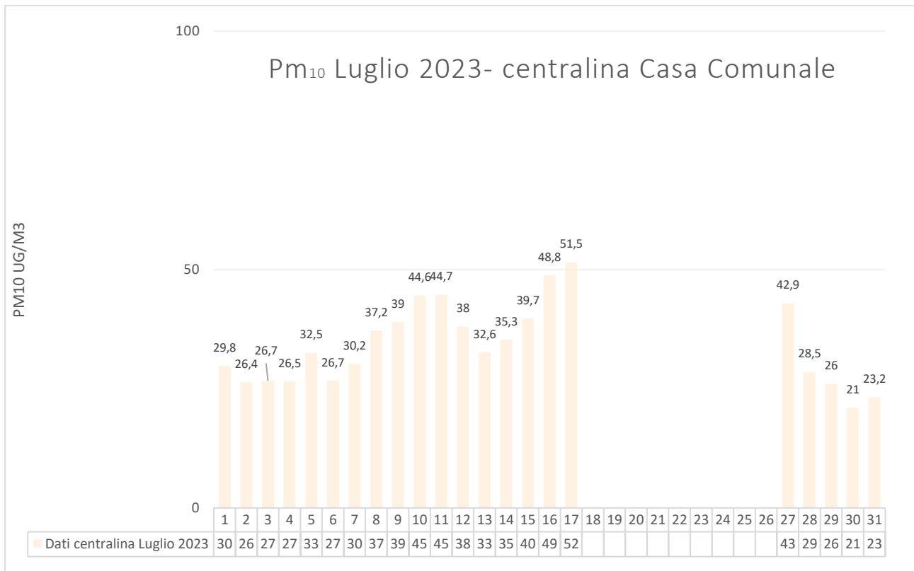
Grafico 1. Andamento polveri sottili PM10 mese di Luglio 2023- Valori rilevati dalla centralina posizionata presso la Casa Comunale (Gestione Ufficio Ambiente)
