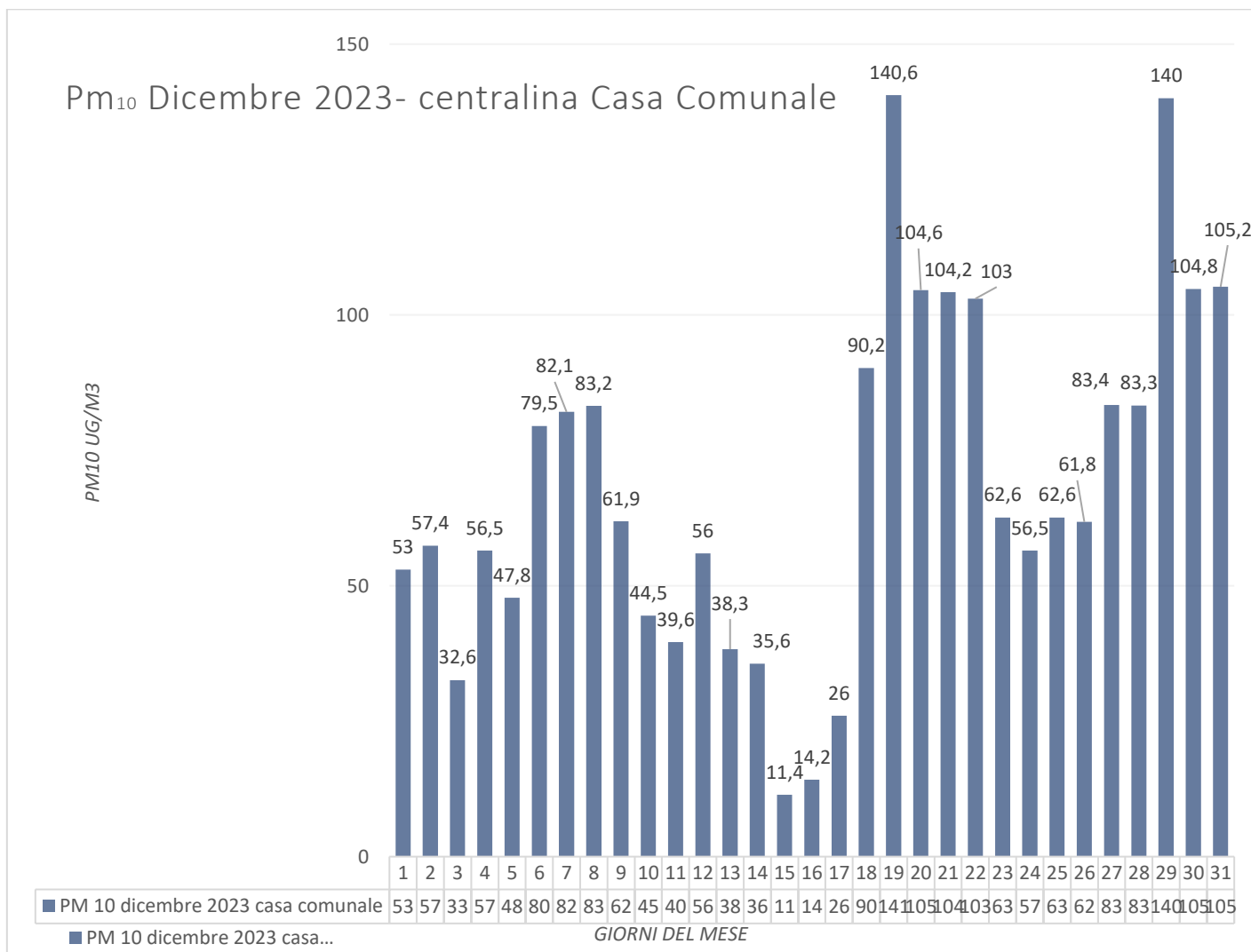
Grafico 1. Andamento polveri sottili PM10 mese di Dicembre 2023- Valori rilevati dalla centralina posizionata presso la Casa Comunale (Gestione Ufficio Ambiente)
