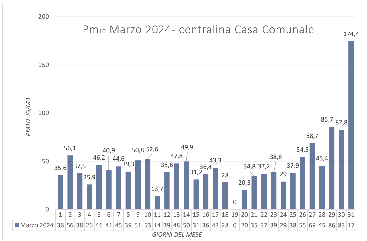
Grafico 1. Andamento polveri sottili PM10 mese di Marzo 2024- Valori rilevati dalla centralina posizionata presso la Casa Comunale (Gestione Ufficio Ambiente)
